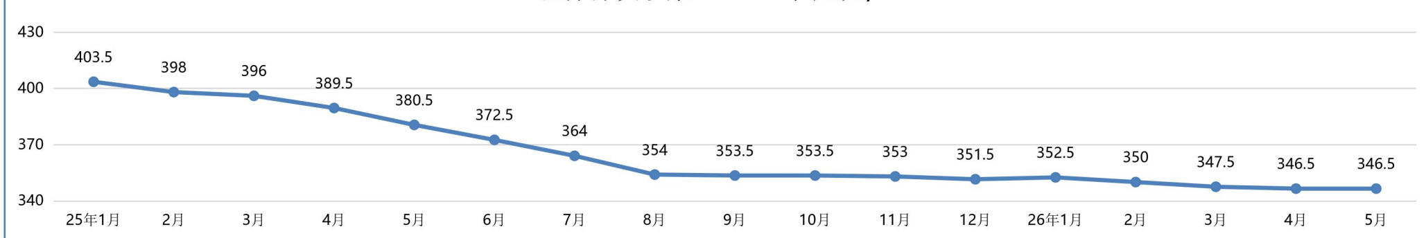
湿拌抹灰砂浆 M20 单位:元/m³
