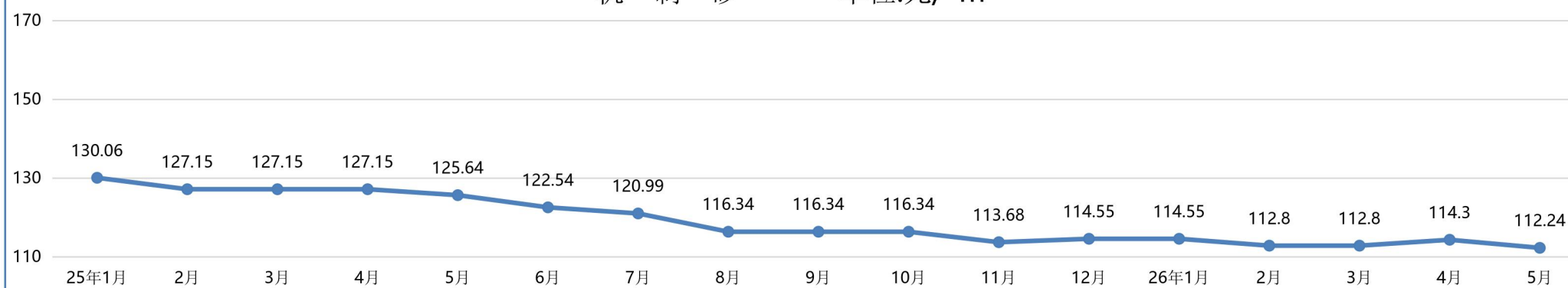
碎 石 10--20 单位:元/m 3
